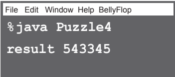
Output
